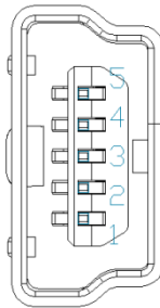
Figure 5: Mini USB Connector
